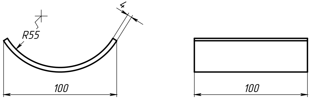
Поз.3 (Ложемент)
