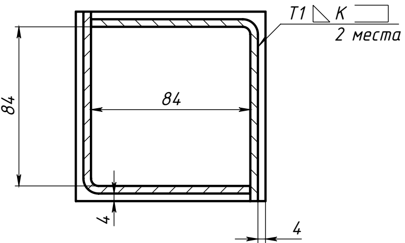
A-A
