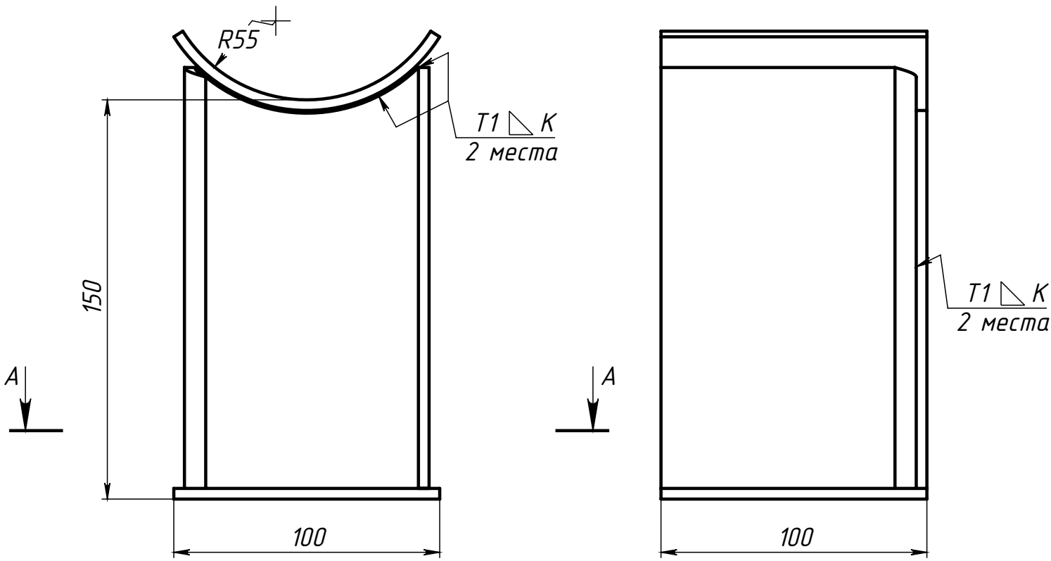
Поз.3 (Ложемент)
